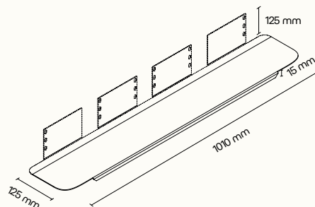
EXTERNE METALL-WANDABLAGE
